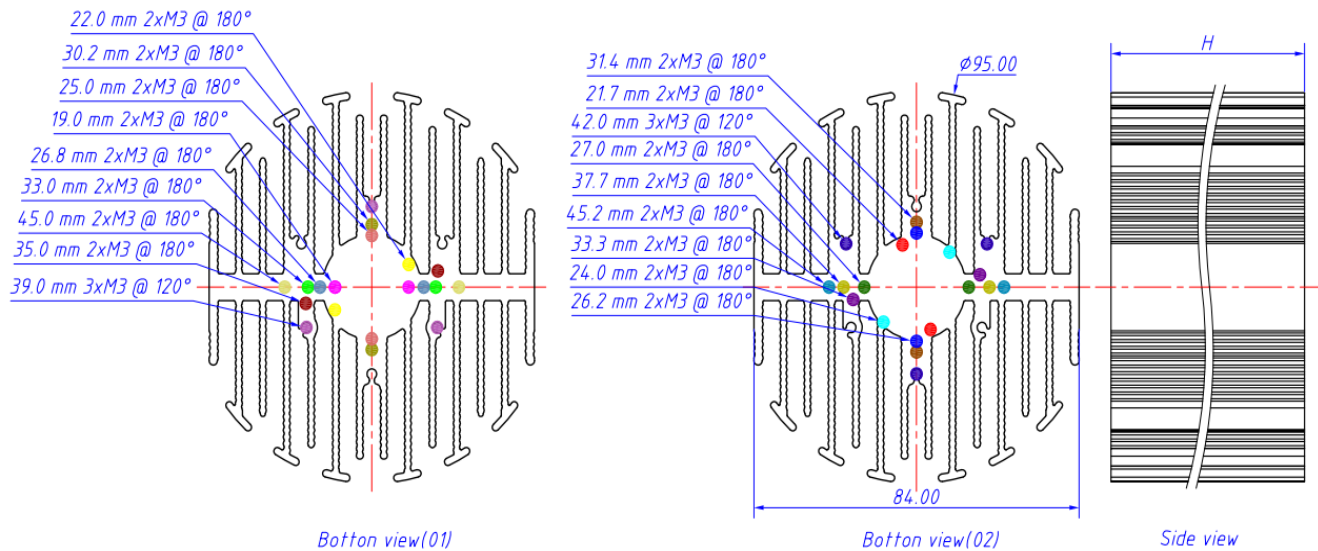
Bottom view(01)
